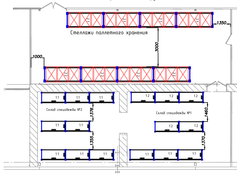
План расстановки оборудования 2D
