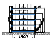
1.1 Стеллаж среднегрузовой (полочный) серии РП50 с разделителями
