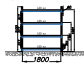
1.2 Стеллаж среднегрузовой (полочный) серии РП50
