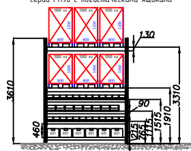
1.2 Стеллаж среднегрузовой (полочный) серии РП50
