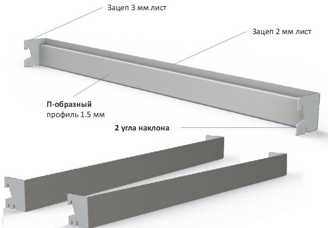
Кронштейн навесной усиленный (ШхГхВ) 906 x 70 x 75 Нагрузка до 70 кг. Вес 3 кг.
