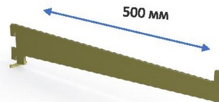
Консоль 500 мм Нагрузка : 40 кг
