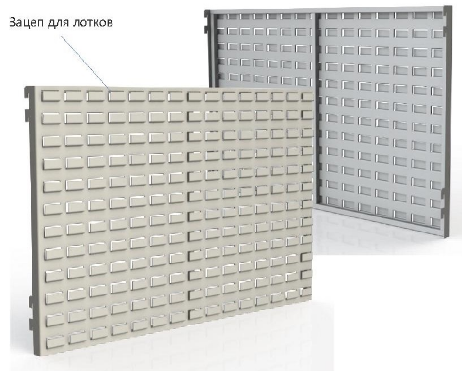
Перфорированная панель для лотков (ДхШхГ) 906 x 586 x 42 Нагрузка на зацеп 15 кг.
