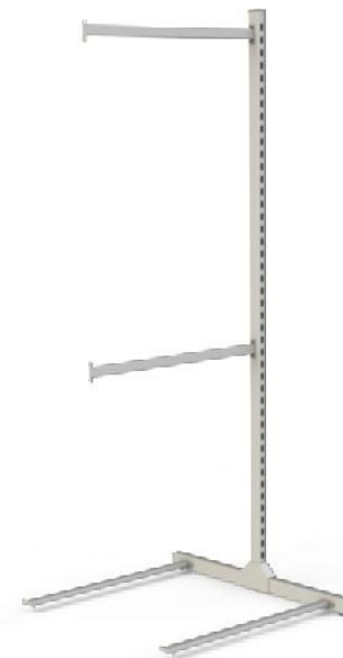
Доп. секция 2-х сторонняя 2400 мм Нагрузка до 1300 кг. (ШхГхВ) 910 x 1008 x 2376 мм
