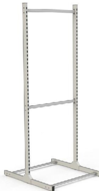
Стойка 2-х сторонняя 2400 мм Нагрузка до 1300 кг. (ШхГхВ) 950 x 1008 x 2376 мм
